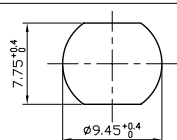
FC Round Adapter DD Style
